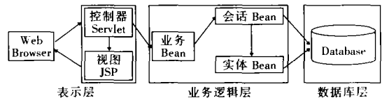
图 2 MVC 模式构筑的 J2EE 平台
