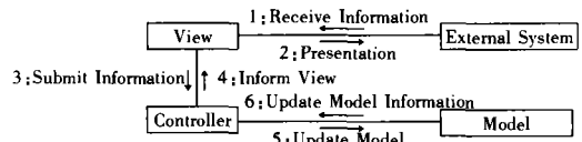
图 1 MVC 模式
